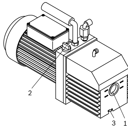
Abb. 24: Vakuumpumpe
