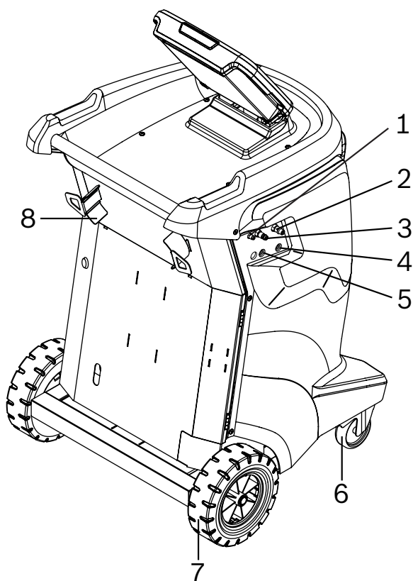
Abb. 2: Rückansicht ACS 753
