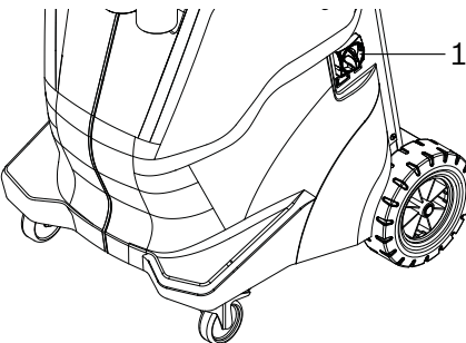
Abb. 21: Hauptschalter
