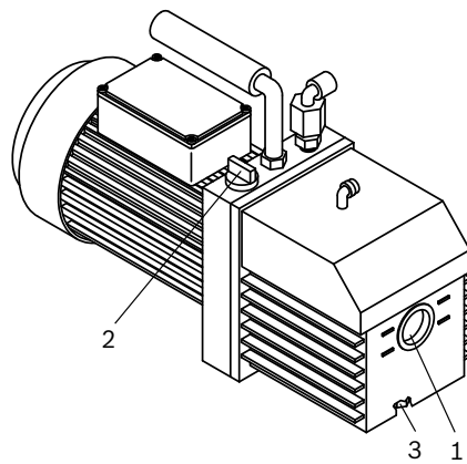
Fig. 24: Bomba de vácuo
