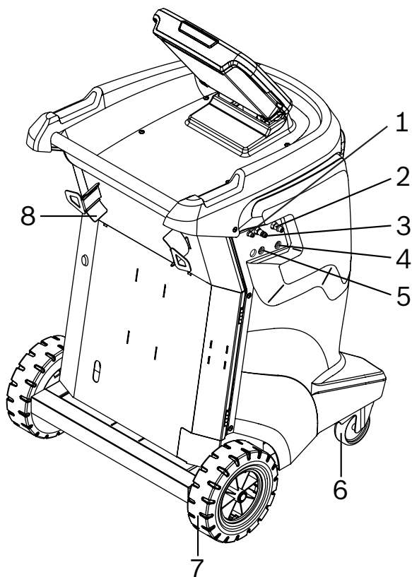
Fig. 2: ACS 753 1 Puerta entrada N2H2 o N2 máx. 14 bar (1.4 MPa) 2 Empalme de lavado (alta presión*) 3 Empalme de lavado (baja presión*) 4 Empalme para tubo de servicio (alta presión*) 5 Empalme para tubo de servicio (baja presión*) 6 Ruedas delanteras con freno de estacionamiento 7 Ruedas traseras 8 Soporte enrolla tubos (*) máx. 25 bar (2.5 MPa)
