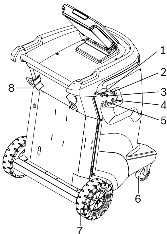
Fig. 2: ACS 753 1 Orifice d'entrée N2H2 ou N2 max 14 bar (1.4 MPa) 2 Embout de lavage (haute pression*) 3 Embout de lavage (basse pression*) 4 Embout pour tuyau de service (haute pression*) 5 Embout pour tuyau de service (basse pression*) 6 Roues avant avec frein de stationnement 7 Roues arrière 8 Support d'enroulement des tuyaux (*) max 25 bar (2.5 MPa)
