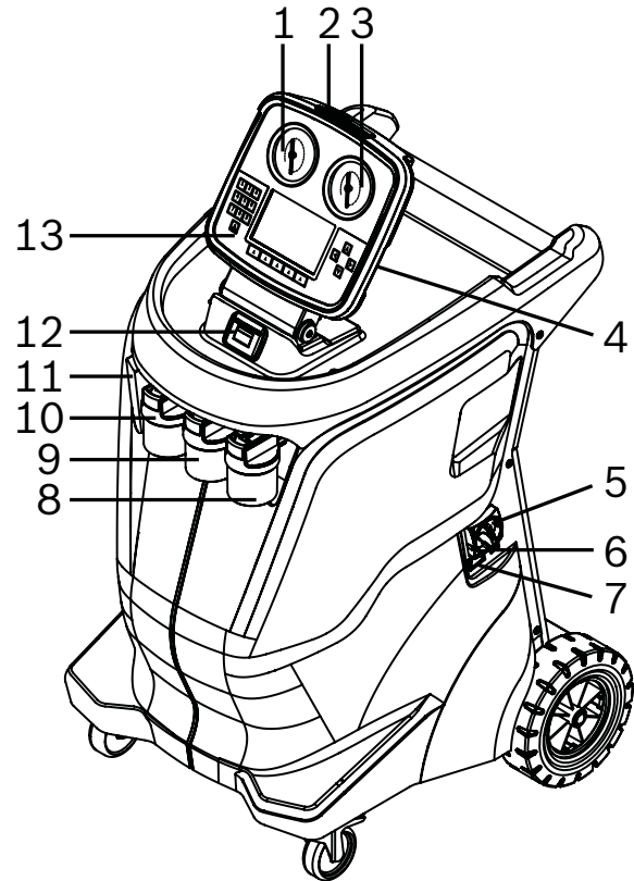
Abb. 1: Vorderansicht ACS 753
