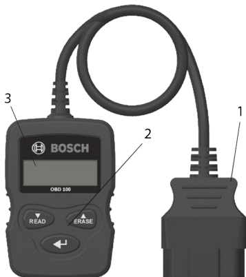
Abb. 1: OBD 100 1 Enchufe para diagnósticos OBD 2 Teclado 3 Pantalla LCD (de dos líneas)
